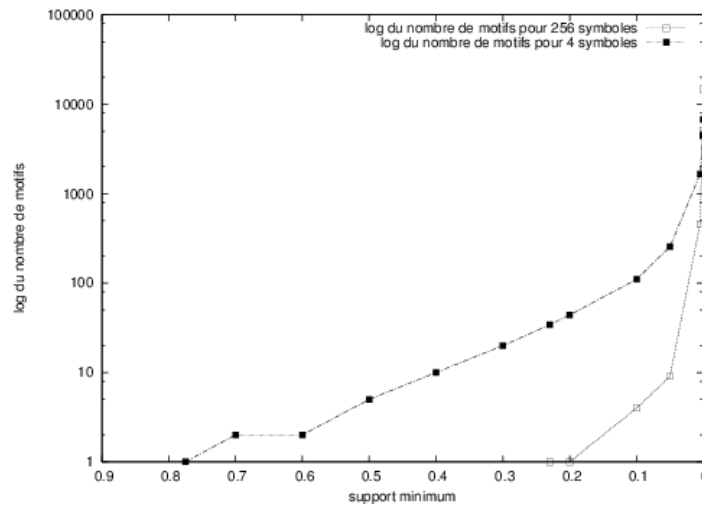
(a) Nombre de motifs en fonction du support minimum (de 0 à 90%).
