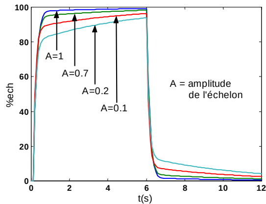
Fig. 10 : Réponse à des échelons d'amplitude différente ( 3 \times 5 règles).
