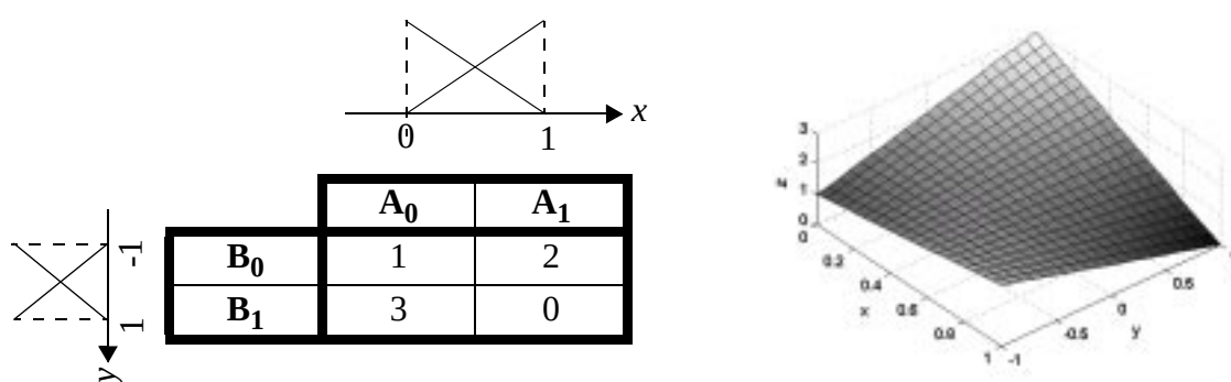
Fig. 23 : Exemple de sous-système flou élémentaire.
